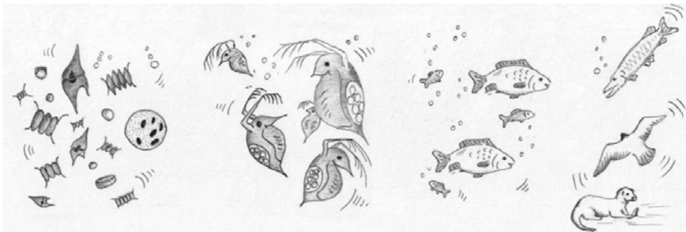
Potravní řetězec rybníka: řasy a sinice (fytoplankton) vytvářejí svá těla fotosyntézou s využitím živin a oxidu uhličitého. Slouží jako potrava zooplanktonu a ten je požírán rybami, které jsou potravou dravých ryb, rybožravých ptáků, vyder i člověka.
